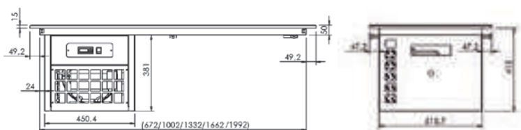
MEDIDAS PLACA FRÍA
