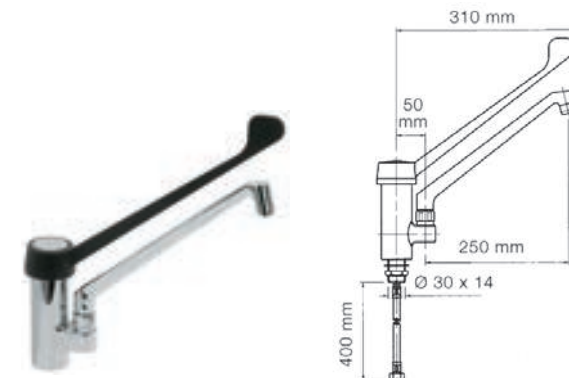
Modelo Grifo de codo gerontológico Código R0020215
