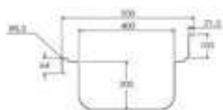
MEDIDAS CUBETA
