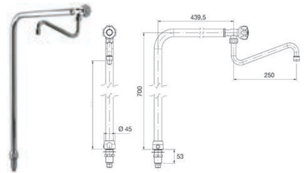
Modelo Grifo columna un agua Código • R0020219
