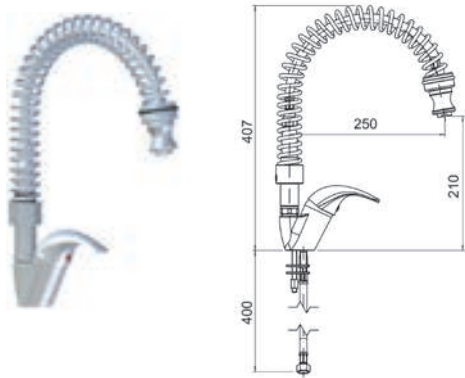
Modelo Grifo mezclador monomando espiral Código • R0020239
