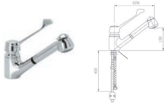
Modelo Grifo mezclador dos aguas con caño extraíble Código • R0020223
