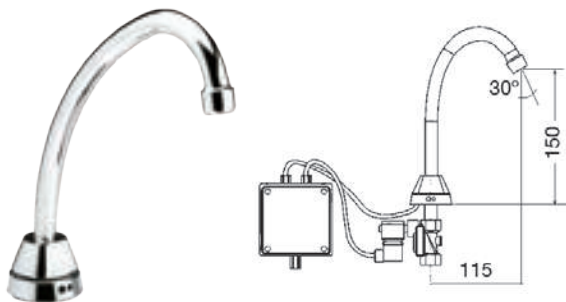
Modelo Grifo electrónico de caño alto a red Código • R0020230
