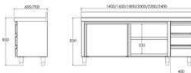
MEDIDAS MUEBLE CON CAJONES Y PUERTAS CORREDERAS
