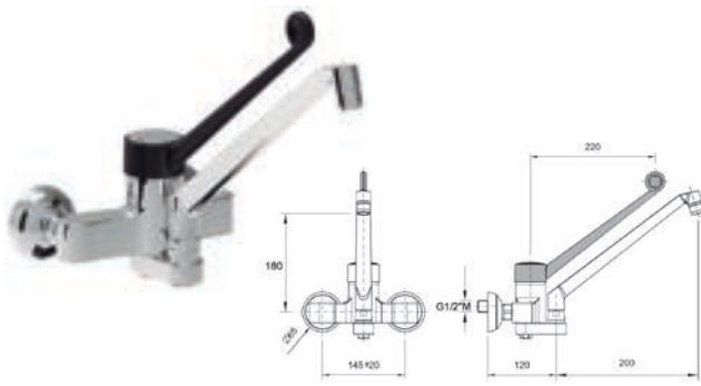
Modelo Grifo mezclador de pared dos aguas Código • R0020222
