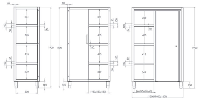
MEDIDAS ARMARIO DE PIE
