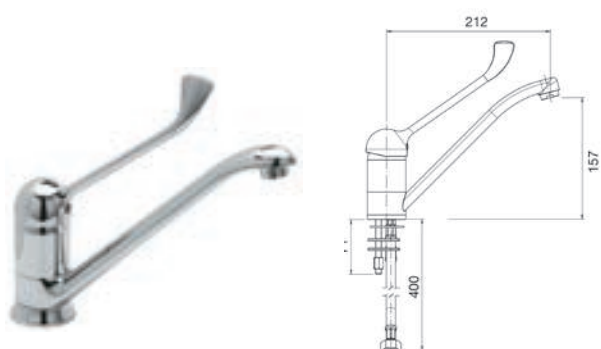
Modelo Grifo caño bajo mando alto Código R0020304
