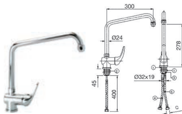
Modelo Grifo caño alto relleno Código R0020238
