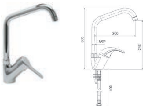
Modelo Grifo caño alto monomando Código R0020202
