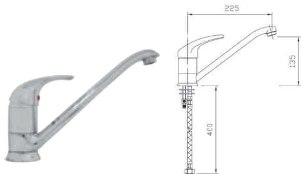
Modelo Grifo caño bajo mando corto Código R0020221
