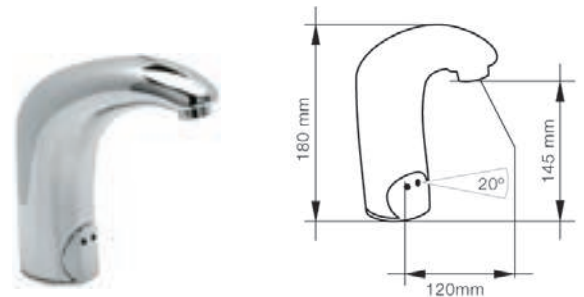
Modelo Grifo electrónico a red Código • R0020214 Grifo electrónico con pilas Código • R0020229
