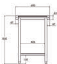
MEDIDAS MESA CENTRAL
